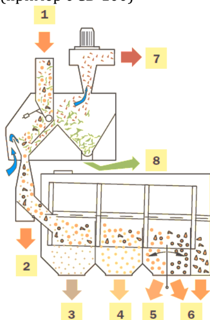
Схема работы (пример с СВ-100)
