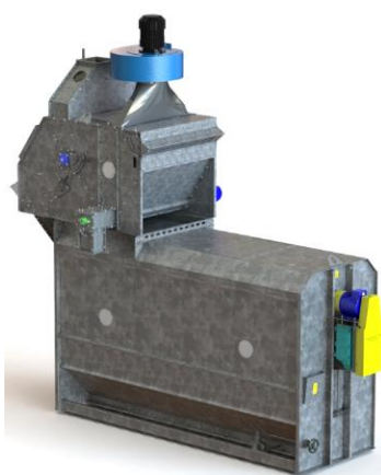
Сепаратор барабанный с СВ-100
